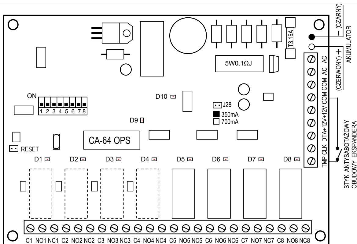
Rysunek 1. Widok płytki ekspandera w wykonaniu „ROC” (4 wyjścia typu OC plus 4 wyjścia przekaźnikowe).
